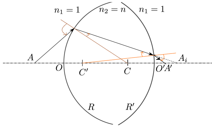
FIGURE 3.2 – Association de deux dioptries sphériques. Sur le dessin, R = \overline{OC} > 0 et R' = \overline{O'C'} < 0 .
